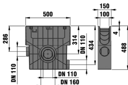
Sumidero con cesta de plástico y reja perforada Ø 6 mm, clase A 15, cerrada
